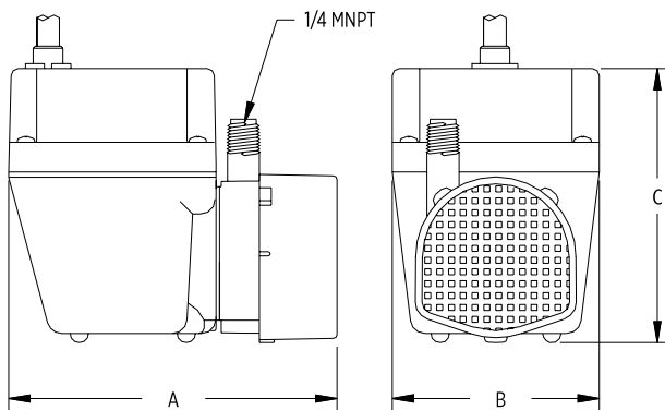
DIMENSIONES (PULG)
